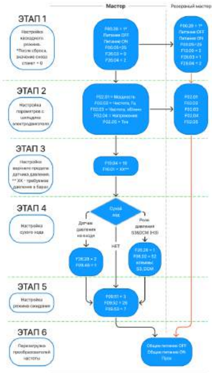
Рис. 12 Пример настройки 2-х насосной станции
