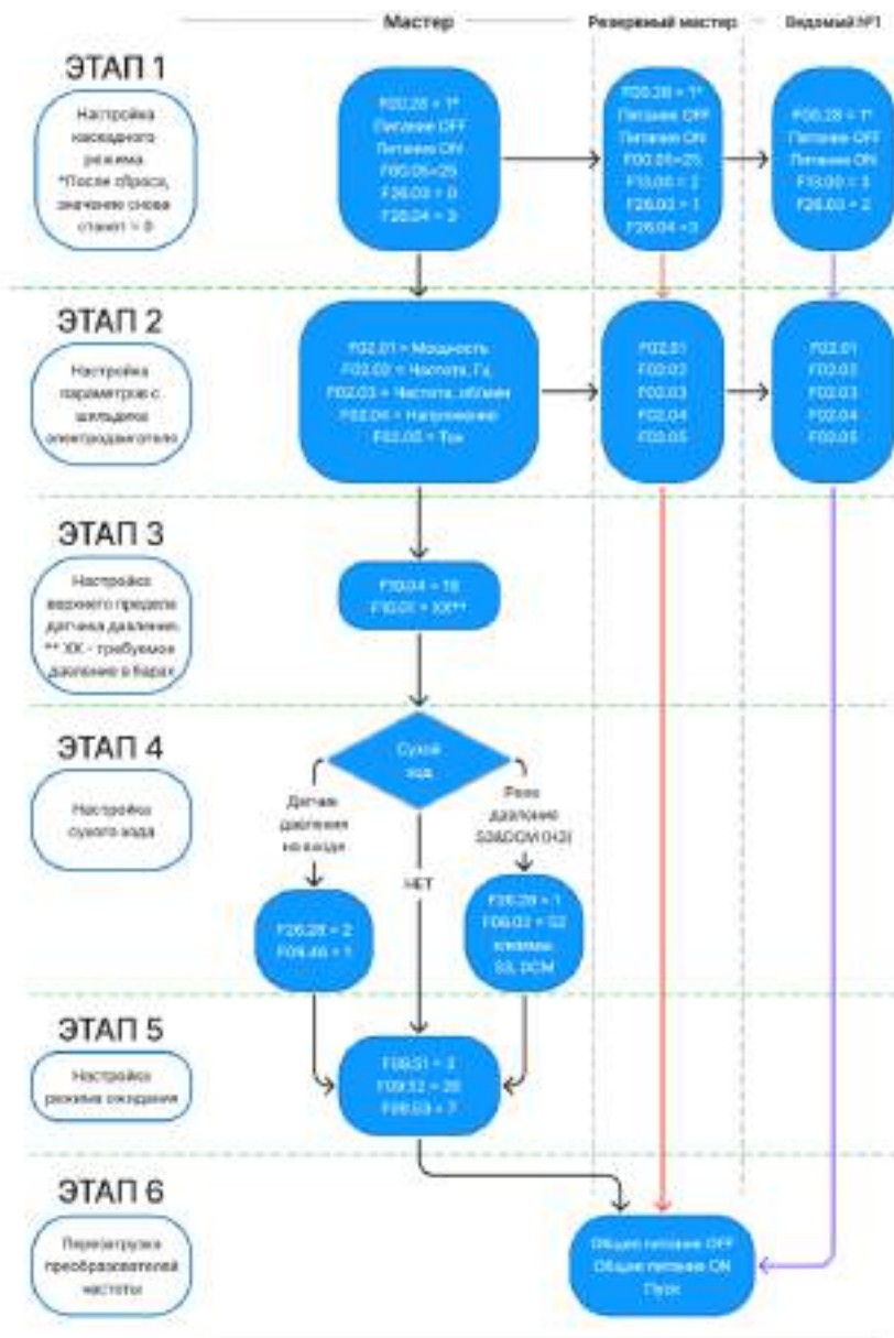
Рис. 13 Пример настройки 3-х насосной станции
