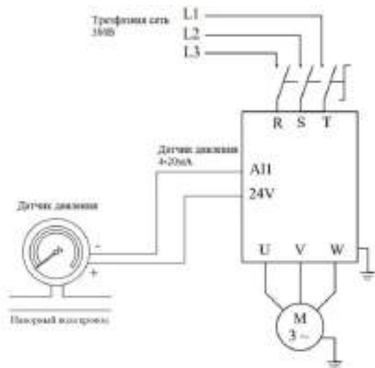
Рис. 10 Схема подключения датчиков
