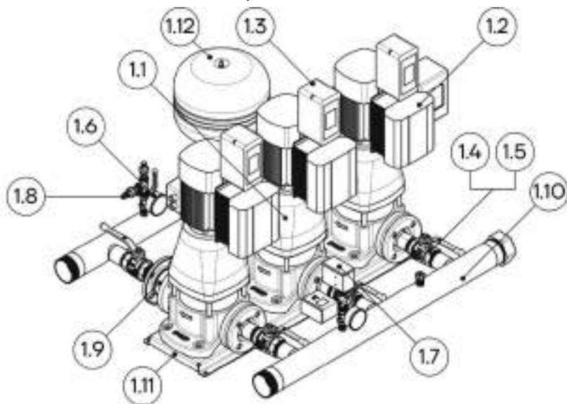
Рис. 1 Внешний вид УПД PBS
