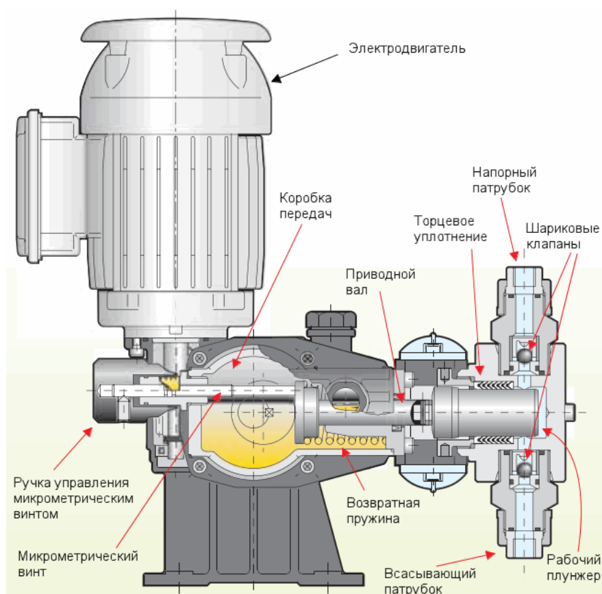
Материалы основных компонентов агрегатов электронасосных дозирующих
