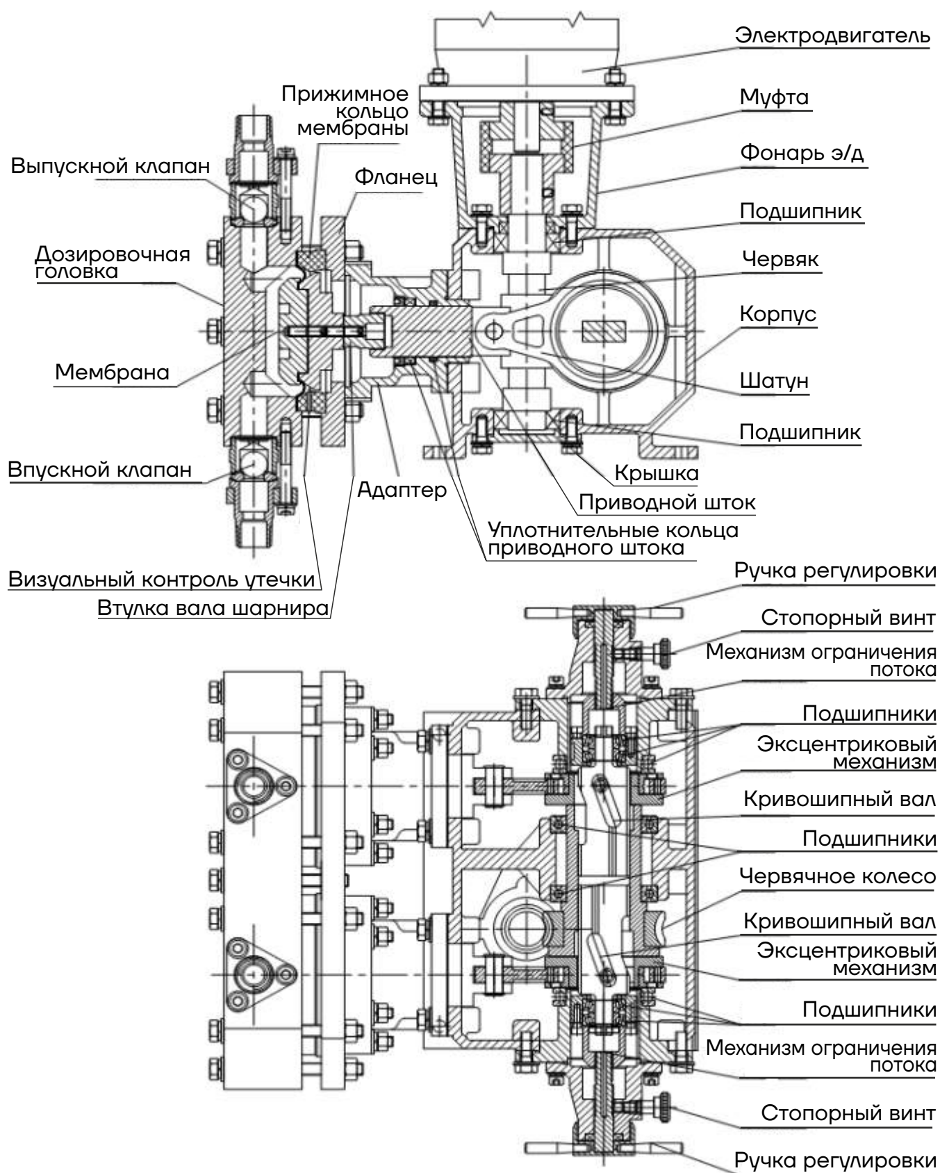
Разрез насоса 2GX
