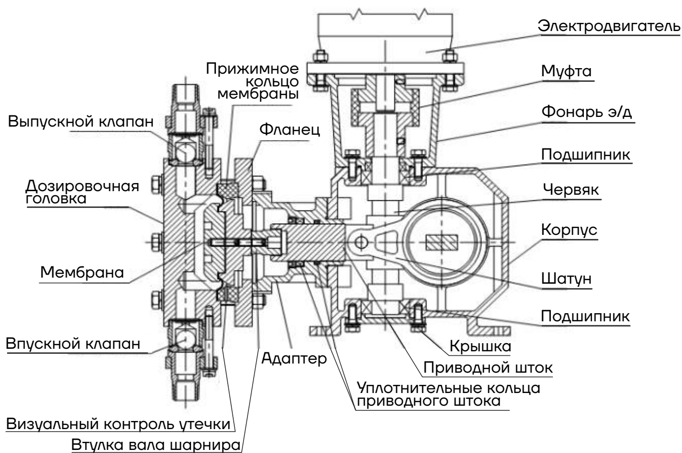
Разрез насоса GX
