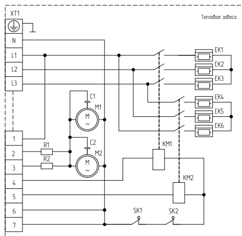
Схема электрическая принципиальная завес ВНС-H20T24-PS, ВНС-H20T36-PS.
