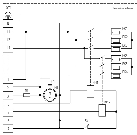
Схема электрическая принципиальная завесы ВНС-H15T18-PS.
