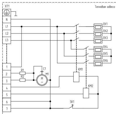
Схема электрическая принципиальная завесы ВНС-H10T12-PS.
