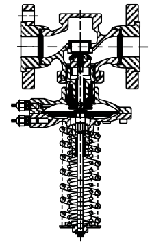
Фланцевое присоединение
